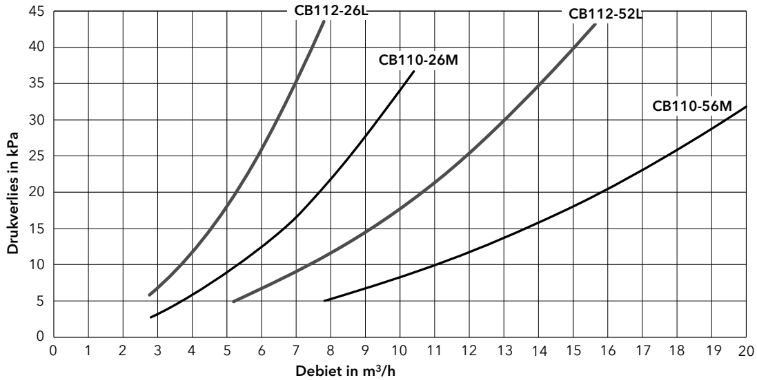
Drukverlies curven Platenwarmtewisselaar voor enkele ketel
