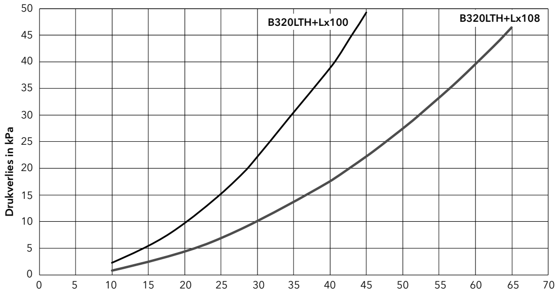
Drukverlies curven Platenwarmtewisselaar voor cascaden
